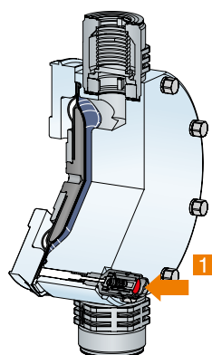
1: Membranbruch-Signalisierung
